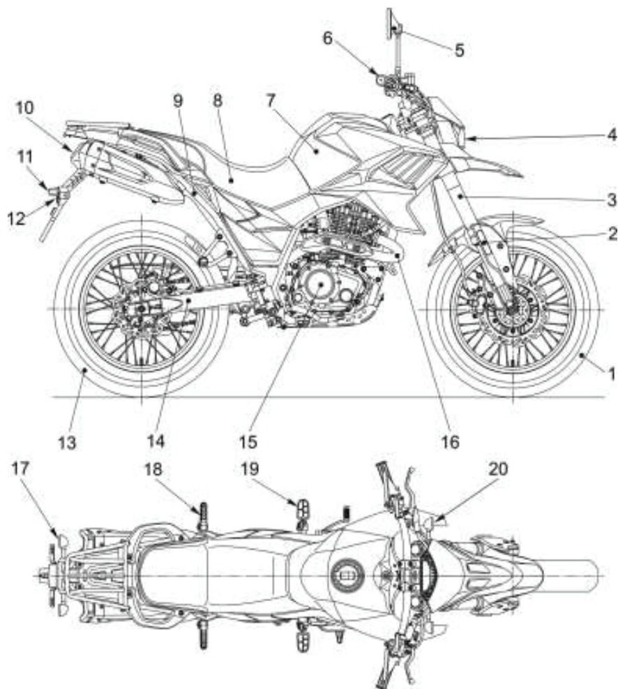
Рисунок 1 – Мотоцикл Tekken 250
