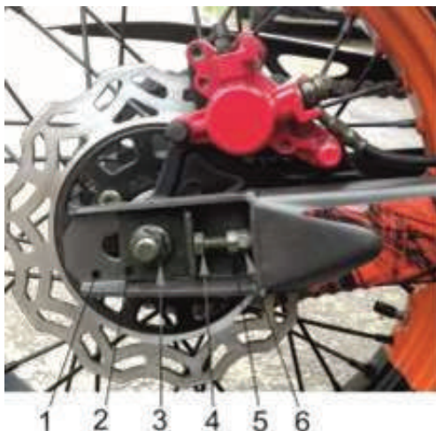
Рисунок 9 – Натяжение цепи
