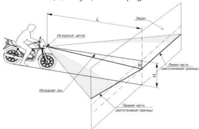
Рисунок 12 – Регулировка светового пучка фары
